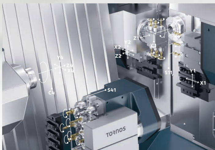
SwissDECO G avec axe A
